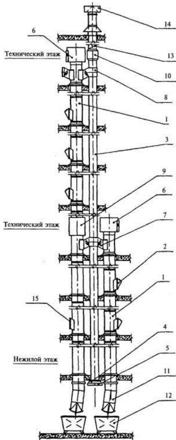
Рисунок 1. Система мусороудаления в высотных зданиях
