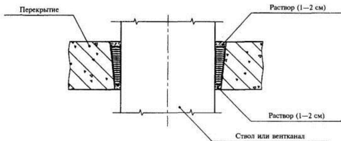
Рисунок 3. Звукоизоляция междуэтажных перекрытий
