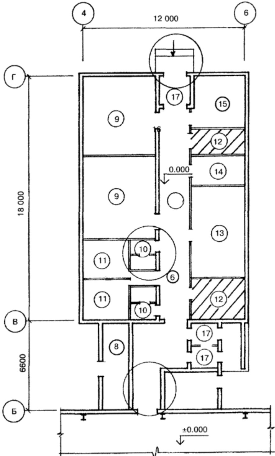
Фрагмент плана на отм. 0.000
