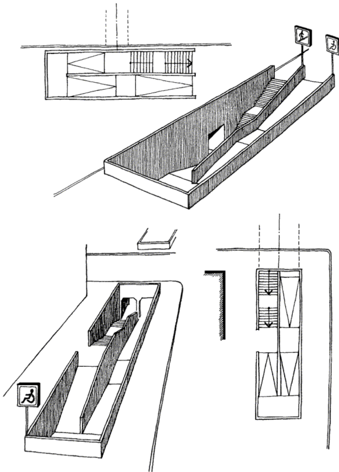
Рисунок 16 - Устройство подземных переходов на предзаводской и заводской (на крупных предприятиях) территориях, обеспечивающее передвижение работников с нарушениями опорно-двигательного аппарата
