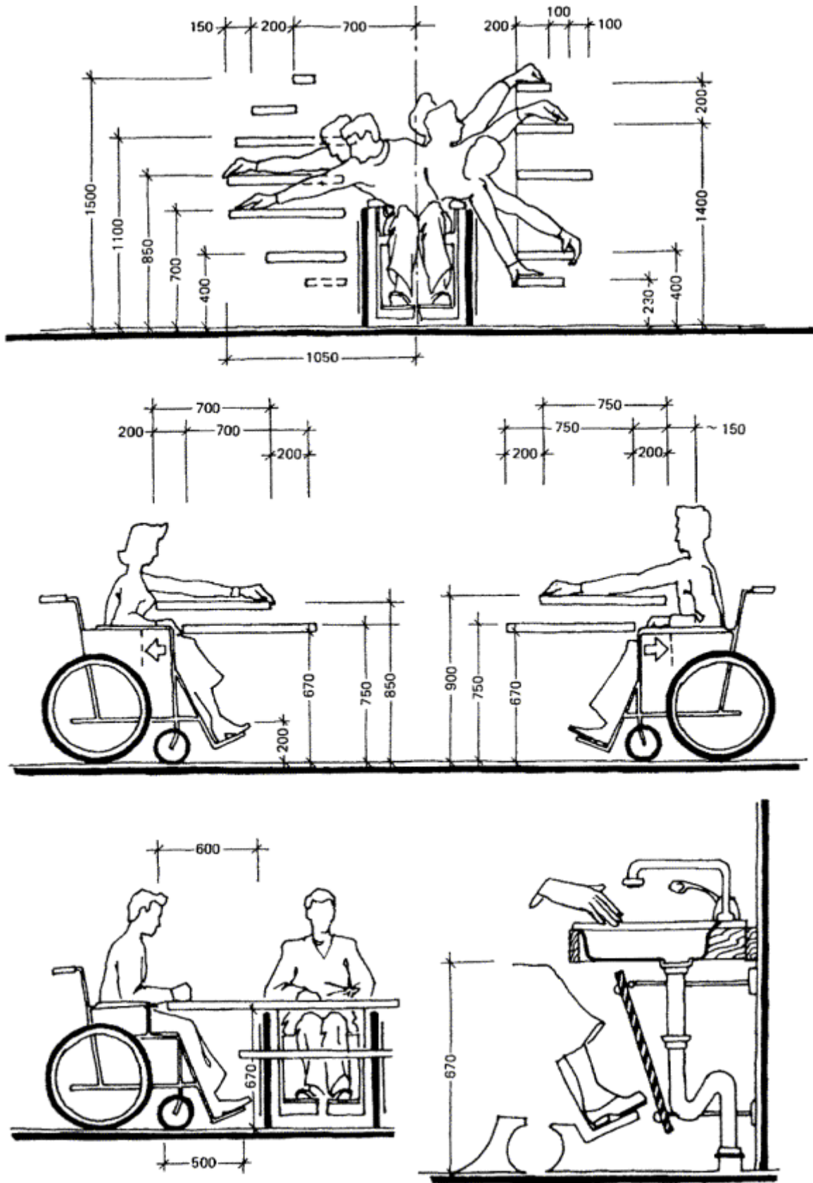
Рисунок 5 - Габариты мебели и оборудования для работника, пользующегося креслом-коляской
