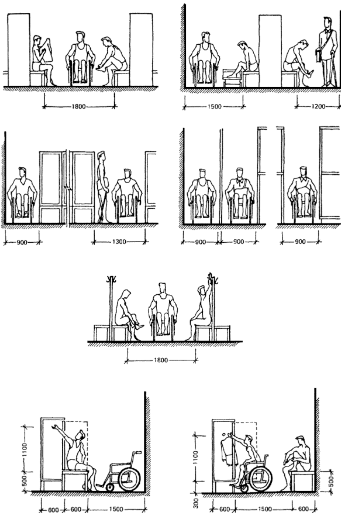
Рисунок 11 - Планировка санитарно-бытовых помещений с учетом работников, имеющих нарушения опорно-двигательного аппарата
