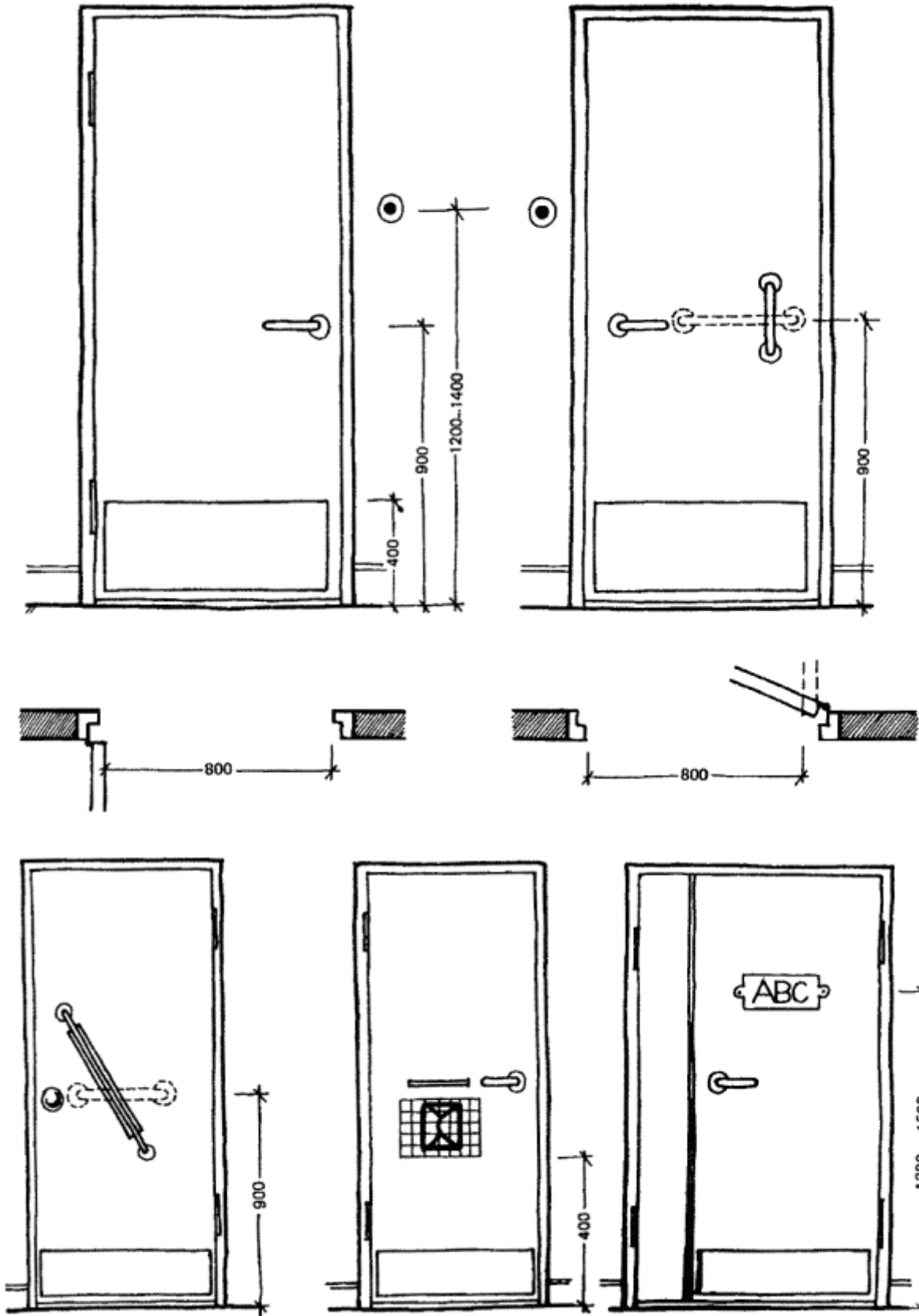
Рисунок 10 - Оборудование дверных проемов
