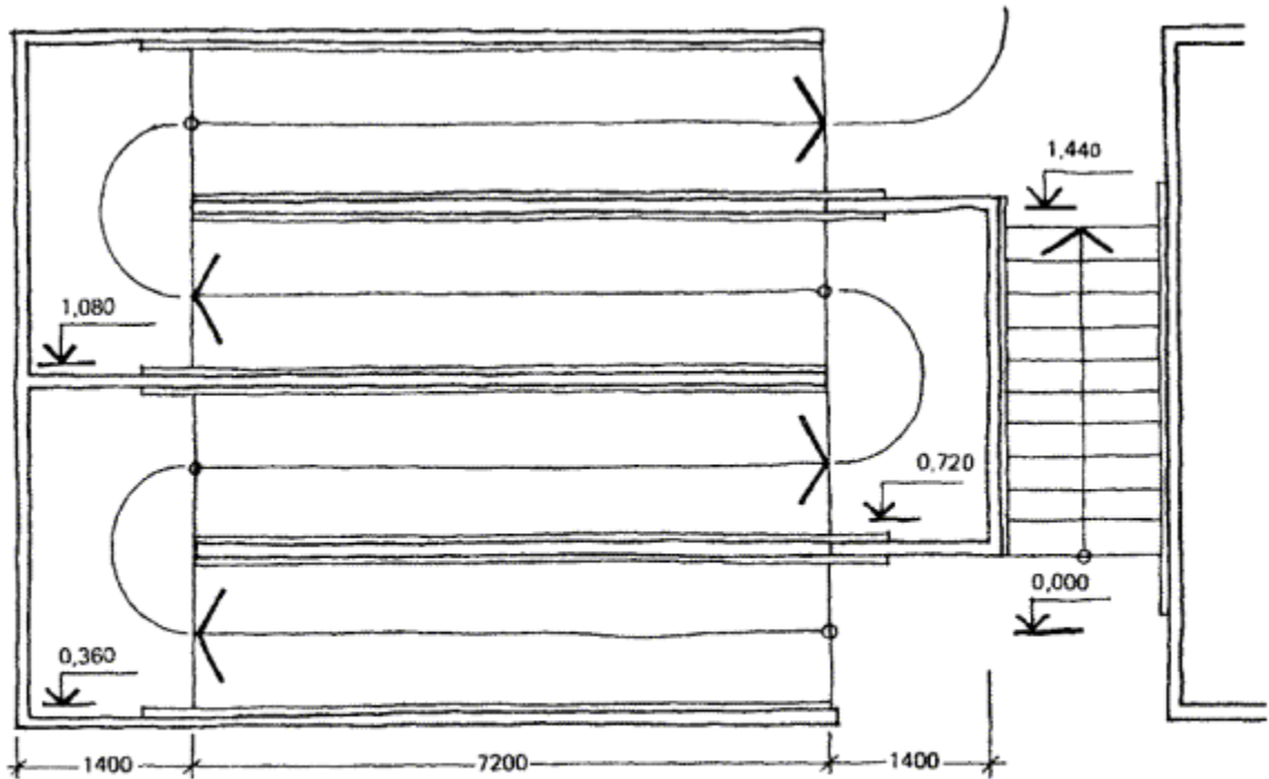
Рисунок 15 - Планировка мест для работников на креслах-колясках в залах питания
