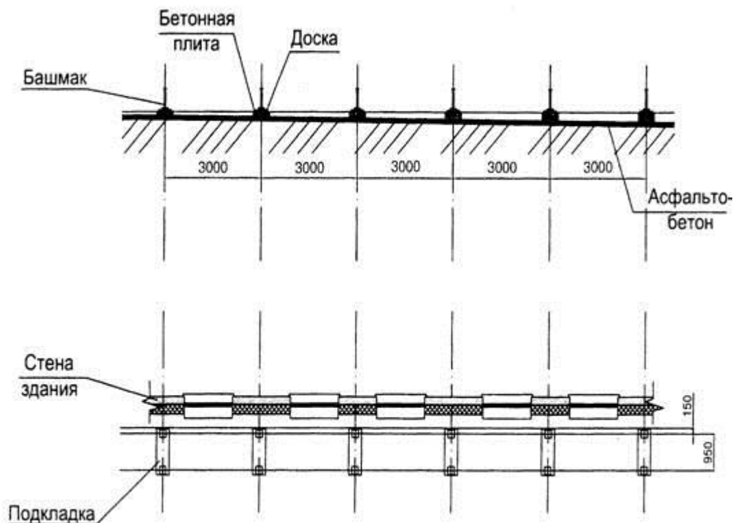
Рис. 3. Установка башмаков
