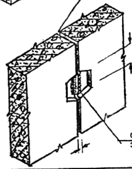
СХЕМА УЗЛОВ СОПРЯЖЕНИЯ ДИАФРАГМ ЖЕСТКОСТИ ПО СЕРИИ I.020-2с
