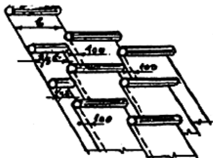
РАСКЛАДКА РУДОННЫХ МАТЕРИАЛОВ ПРИ ТРЕХСЛОЙНОМ КРОВЕЛЬНОМ КОВРЕ
