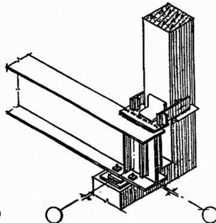
КРЕПЛЕНИЕ СТАЛЬНОЙ ПОДКРАНОВОЙ БАЛКИ
