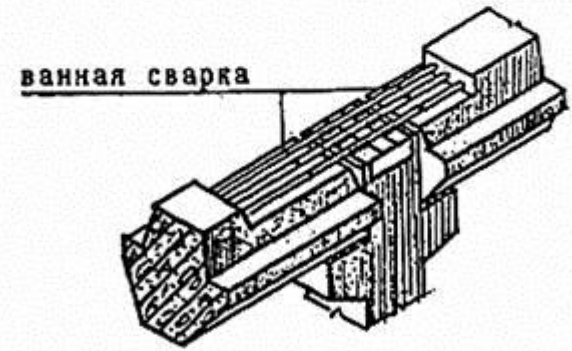
Схема узлов сопряжения ригелей с крайней и средней колоннами в верхнем этаже, у торцов здания и температурных швов
