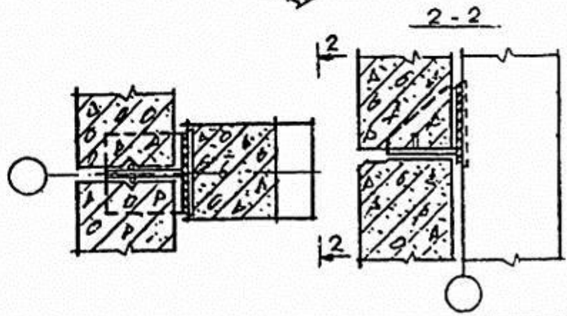
СХЕМА УЗЛОВ КРЕПЛЕНИЯ СТЕНОВЫХ ПАНЕЛЕЙ
