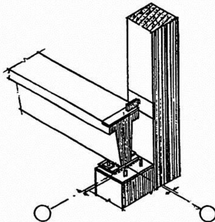
КРЕПЛЕНИЕ ЖЕЛЕЗОБЕТОННОЙ ПОДКРАНОВОЙ БАЛКИ
