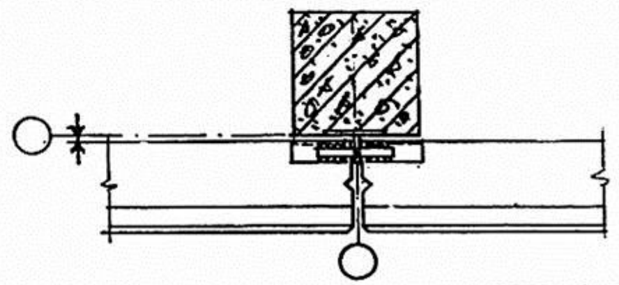
СХЕМА УЗЛА КРЕПЛЕНИЯ ВЕРХА СТЕНОВЫХ ПАНЕЛЕЙ
