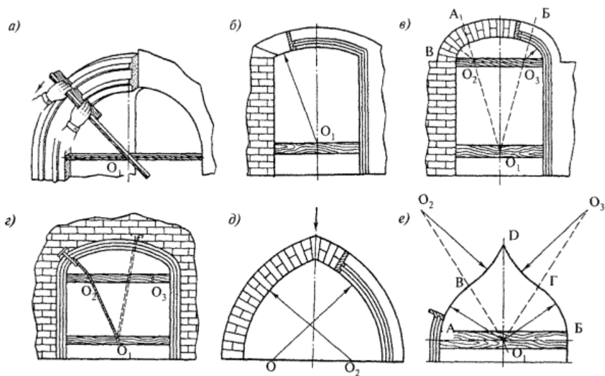
Рис. 26. Вытягивание арок
