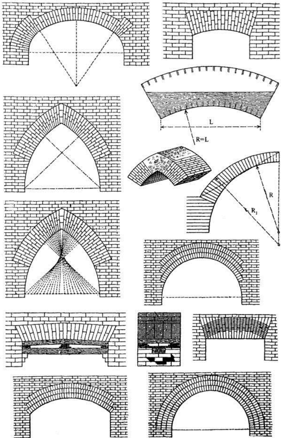
Рис. 46. Кладка арок (из руководства В.Р. Бернгарда, 1901 г.)
