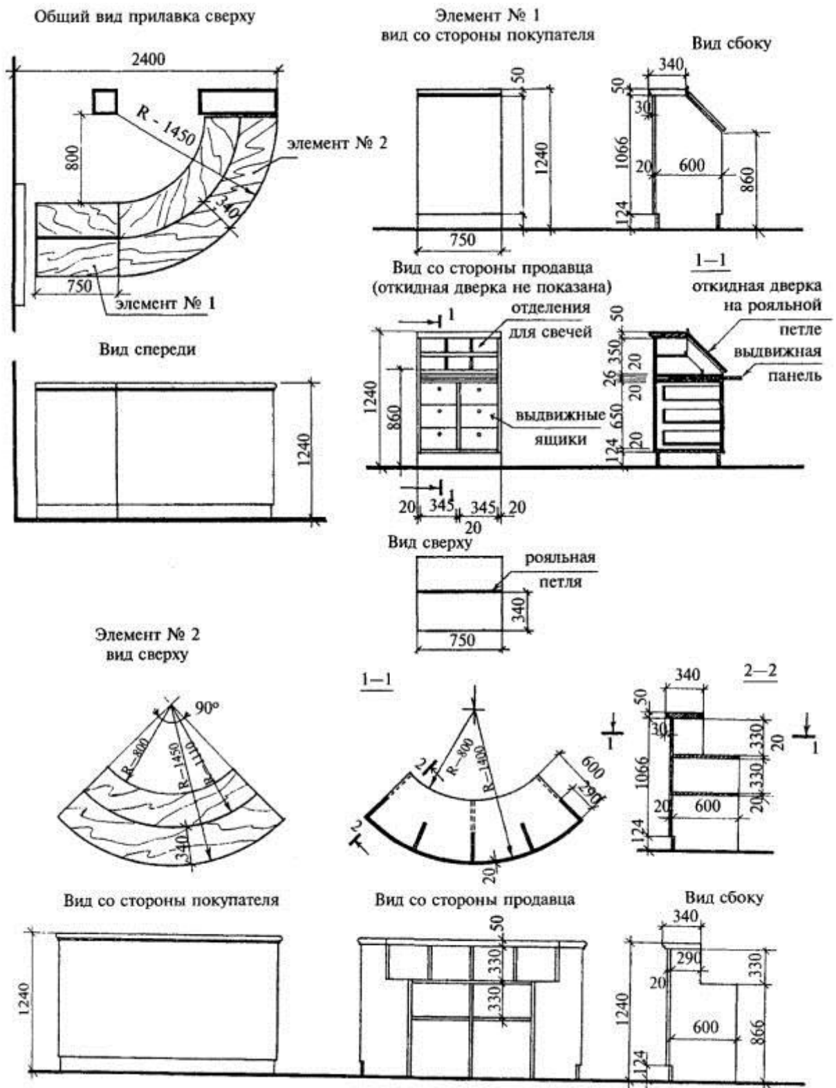
Рис. 40. Свечной ящик (архит. Л. Клешнина)
