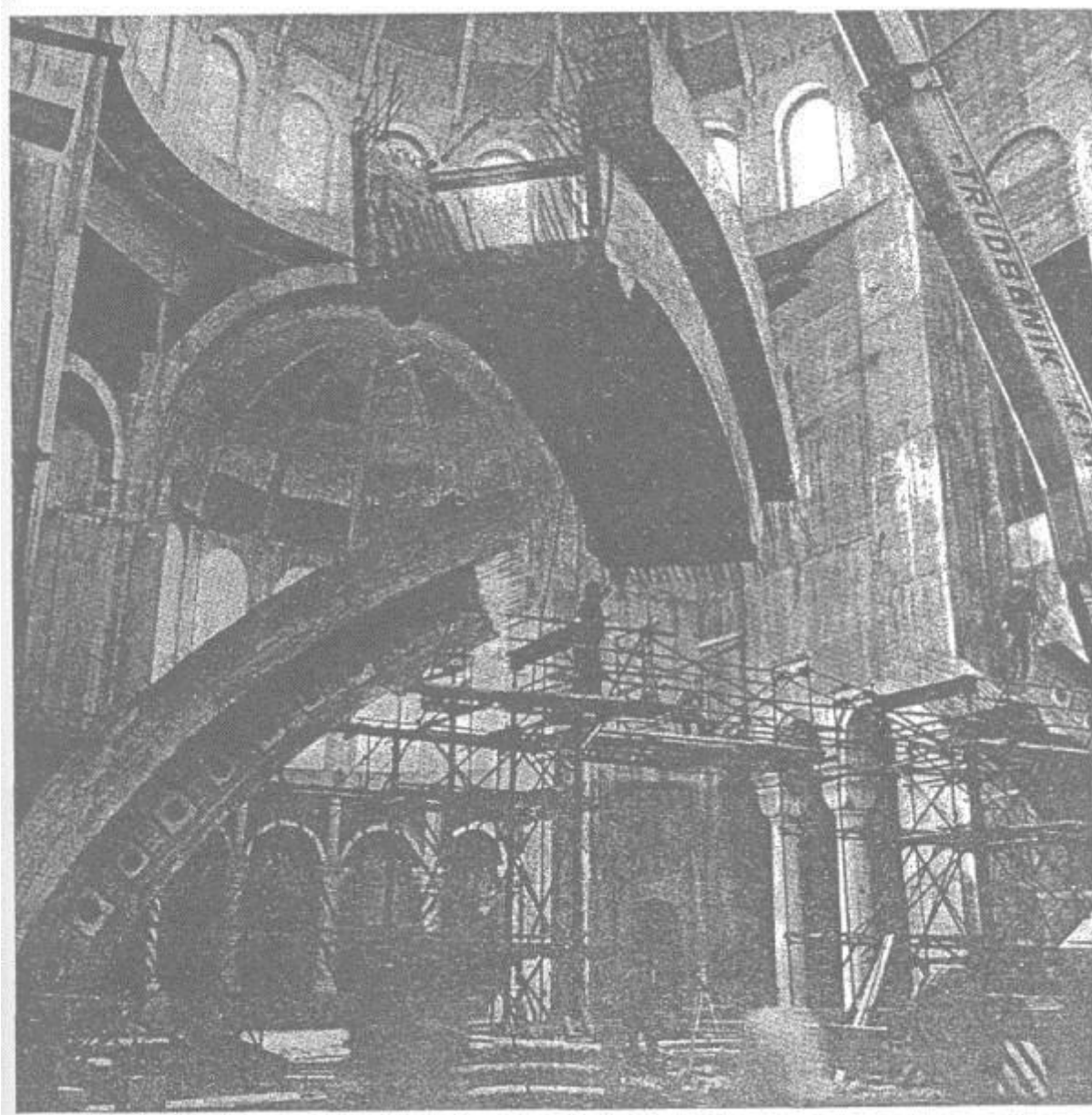
Рис. 60. Подъем конструкций покрытия в соборе св. Саввы в Белграде
