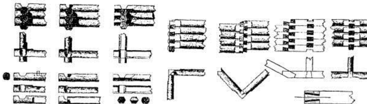
Рис. 52. Конструкции деревянных срубов
