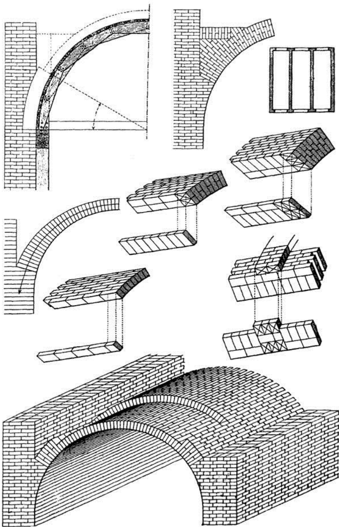
Рис. 49. Кладка сводов (из руководства В.Р. Бернгарда, 1901 г.)
