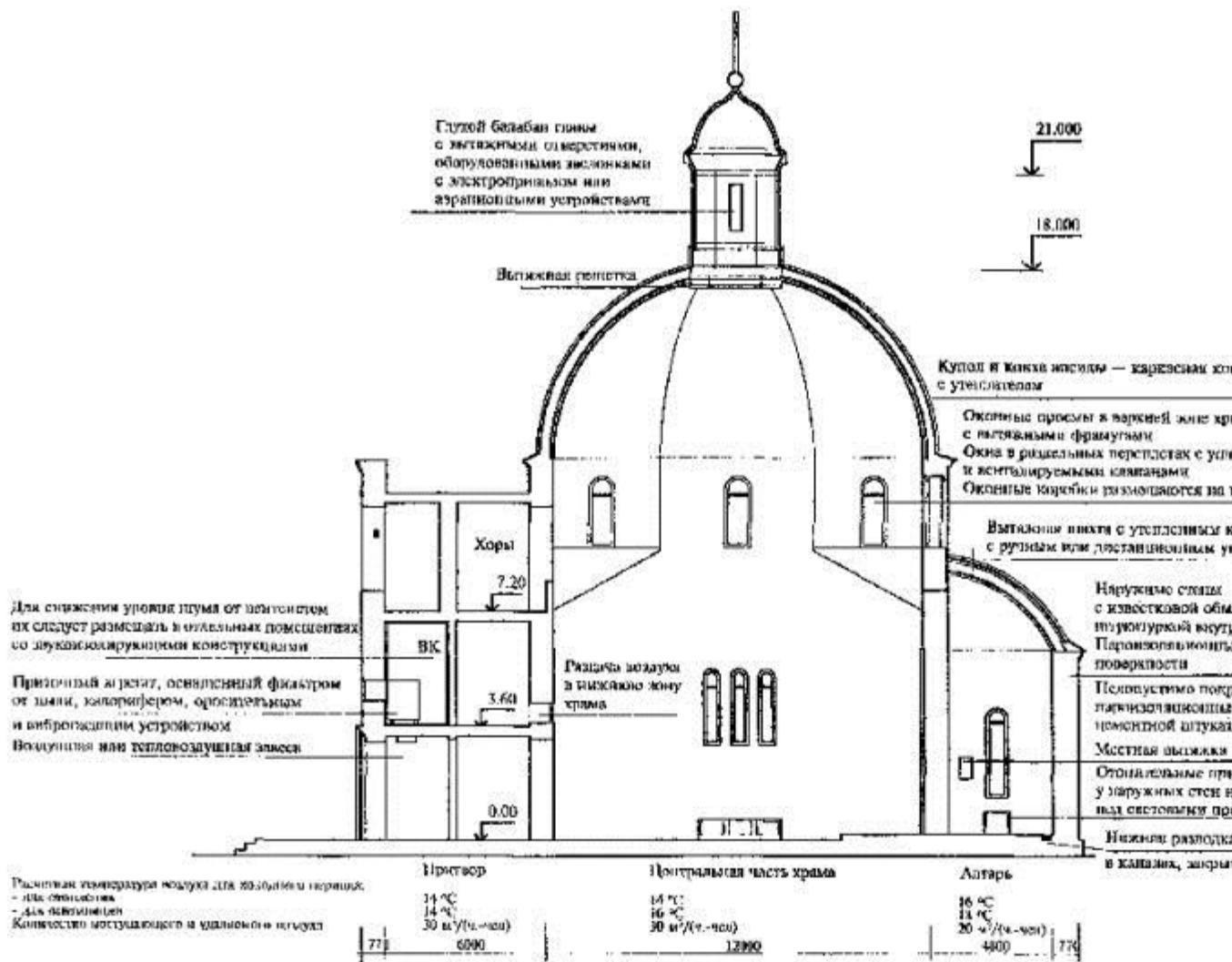
Рис. 61. Схема отопления и вентиляции храма
