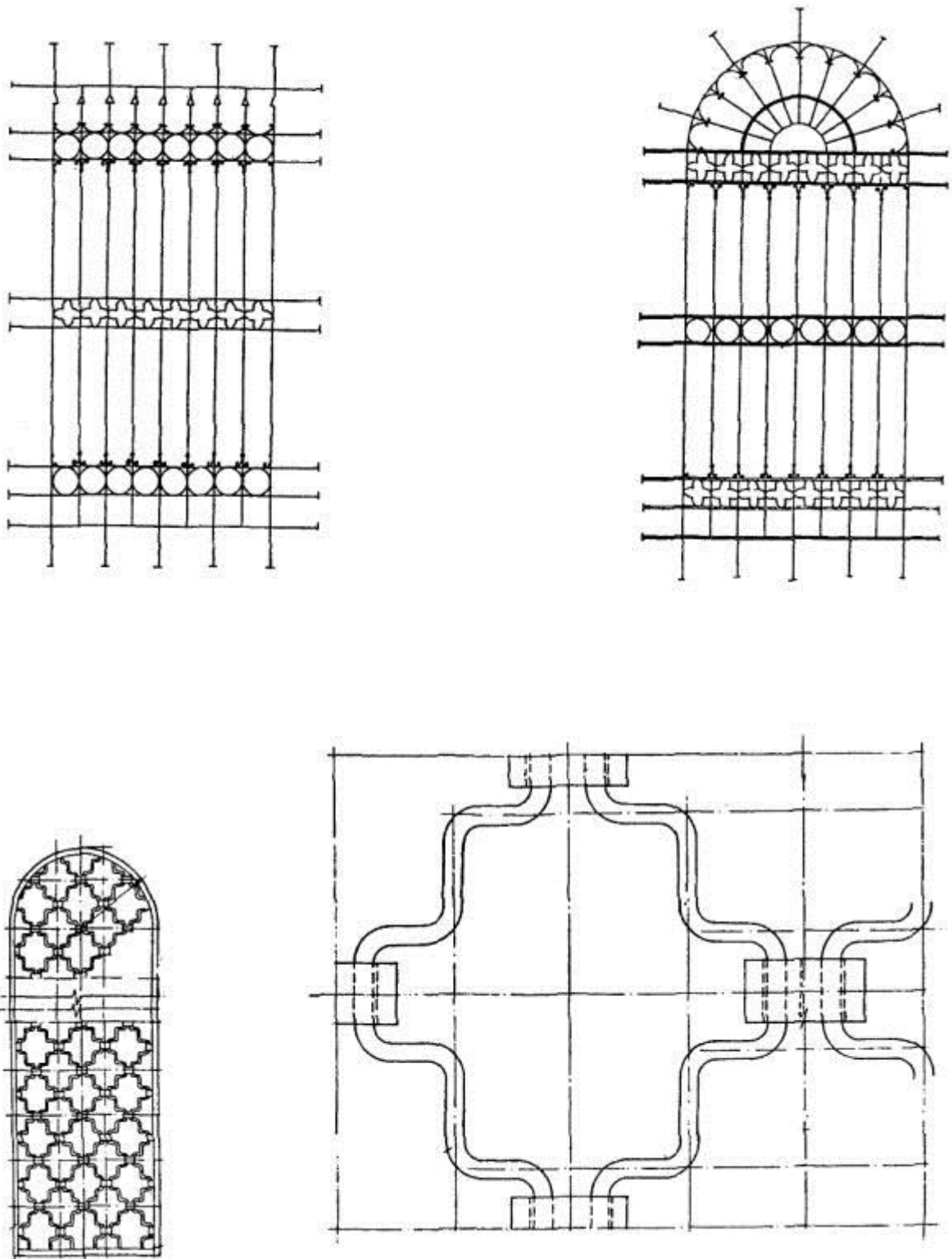
Рис. 21. Оконные решетки
