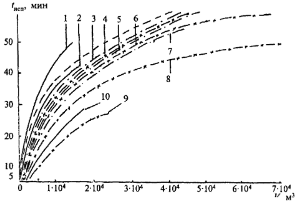
Рис. 4. Зависимость минимальной продолжительности начальной стадии пожара t_{нсн} от объема V , высоты H помещения и количества пожарной нагрузки g
