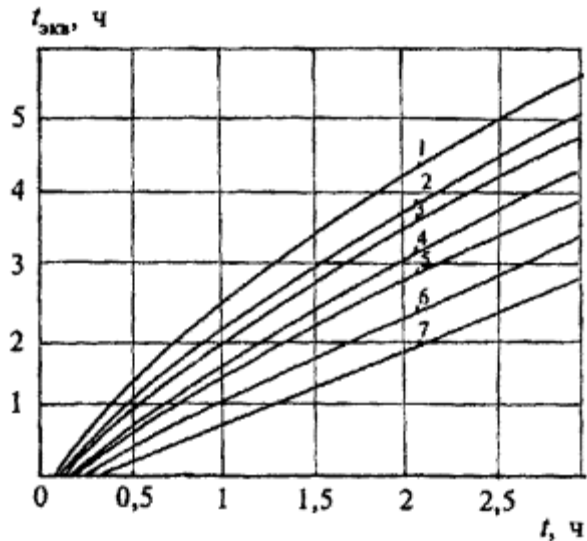
Рис. 8. Зависимость эквивалентной продолжительности пожара для центрально-сжатых железобетонных колонн для ПРВ
