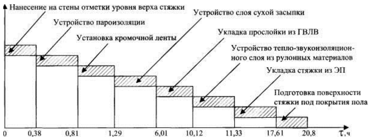
Рис. 6.8.2. График движения рабочей силы при устройстве сборного основания типа «Гамма» по выравнивающему тепло-звукоизоляционному слою сухой засыпки толщиной 60 мм с прослойкой из ГВЛВ на тепло-звукоизоляционном слое из рулонных материалов со стяжкой из элементов пола (к табл. 6.8.2)
