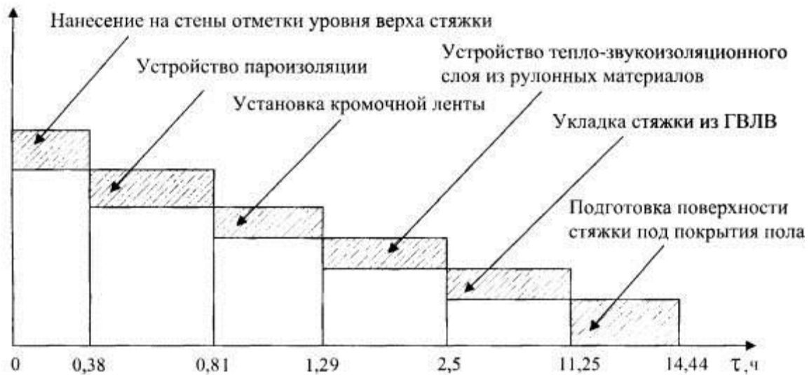
Рис. 6.3.2 а. График движения рабочей силы при устройстве сборного основания типа «Бета» на тепло-звукоизоляционном слое из плитных материалов со стяжкой из малоформатных ГВЛВ (к табл. 6.3.2)
