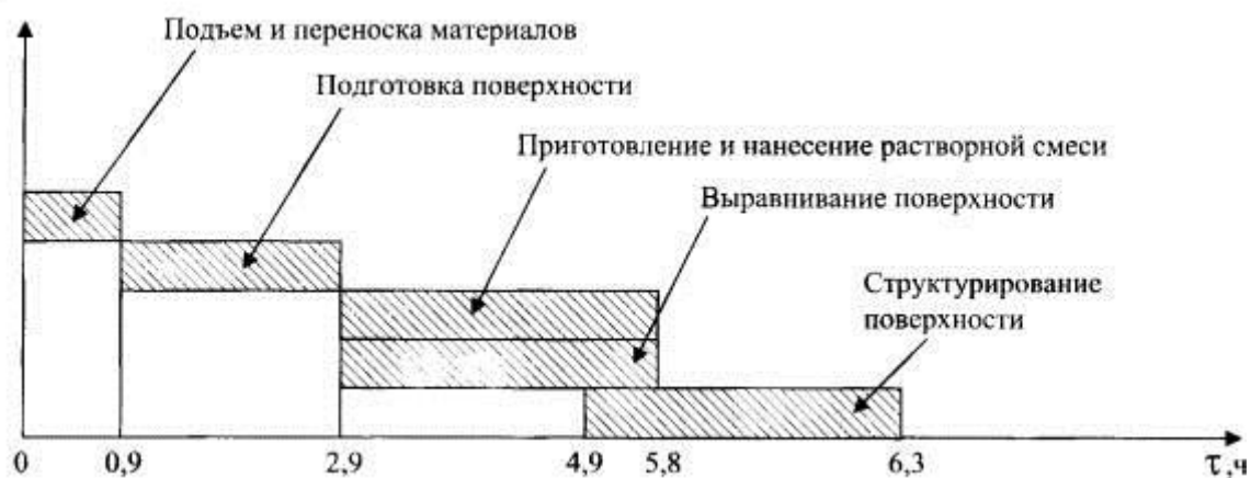
Рис. 6.2. График движения рабочей силы (к табл. 6.8).
