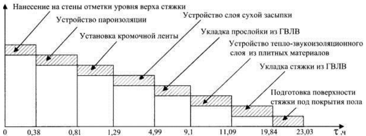
Рис. 6.7.1 а. График движения рабочей силы при устройстве сборного основания типа «Гамма» по выравнивающему тепло-звукоизоляционному слою сухой засыпки толщиной 40 мм с прослойкой из ГВЛВ на тепло-звукоизоляционном слое из плитных материалов со стяжкой из ГВЛВ (к табл. 6.7.1)
