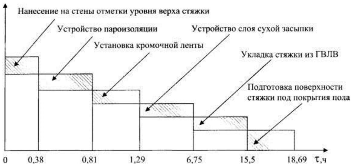
Рис. 6.8 а. График движения рабочей силы при устройстве сборного основания типа «Вега» по выравнивающему тепло-звукоизоляционному слою сухой засыпки толщиной 80 мм со стяжкой из гипсоволокнистых листов влагостойких (к табл. 6.8)
