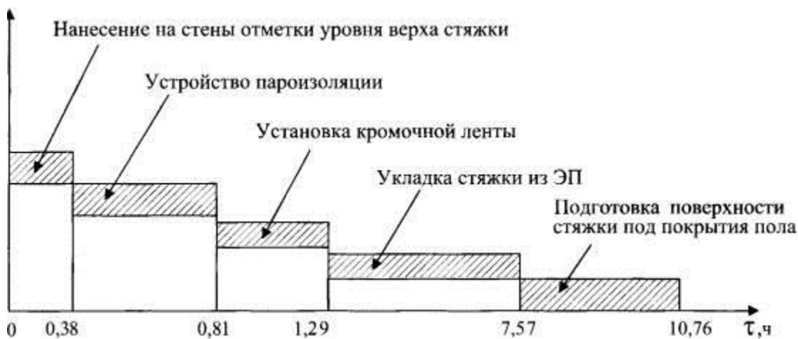
Рис. 6.3. График движения рабочей силы при устройстве сборного основания типа «Альфа» из элементов пола (к табл. 6.3.1)
