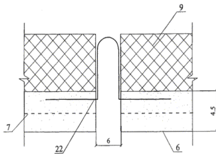
Вариант с поверхностным сбросом дождевой воды
