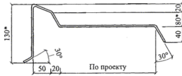
УГЛОВОЙ КОМБИНИРОВАННЫЙ ПРОФИЛЬ
