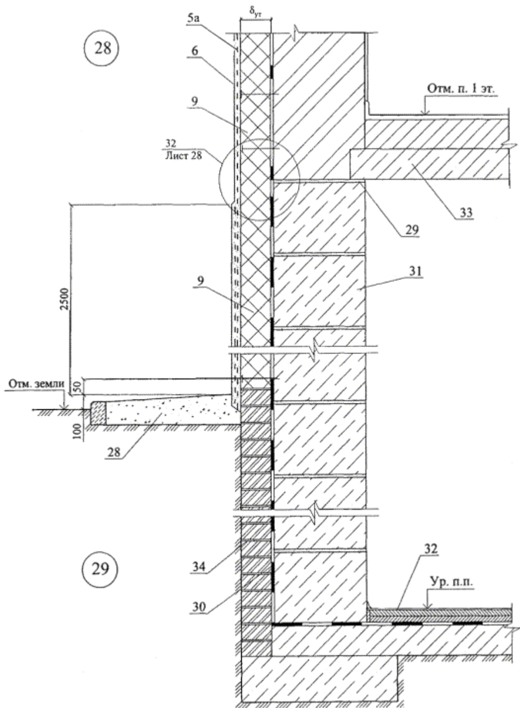
Вариант с дренажем
