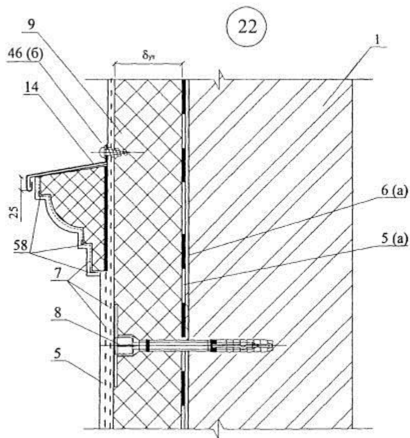
СХЕМА ПРИВЯЗКИ ДЮБЕЛЕЙ
