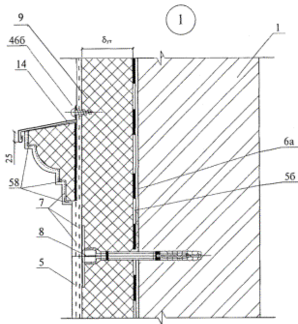
СХЕМА ПРИВЯЗКИ ДЮБЕЛЕЙ
