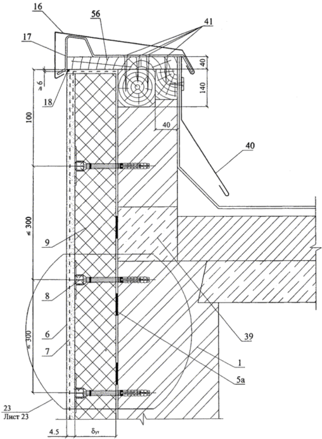
Вариант примыкания с опорным профилем
