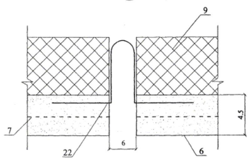
Вариант с поверхностным сбросом дождевой воды
