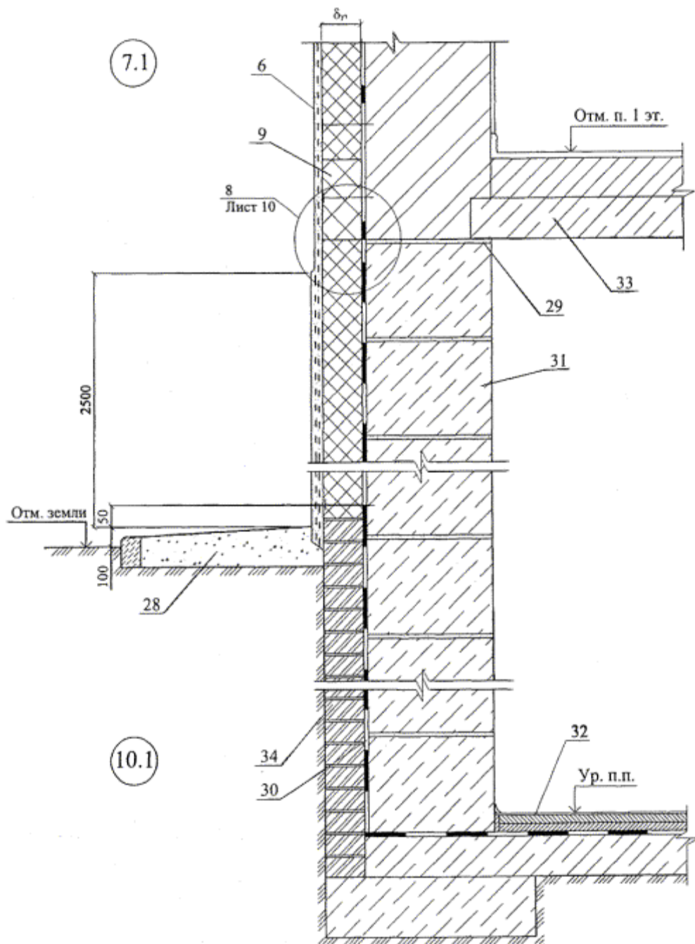
Вариант с дренажем
