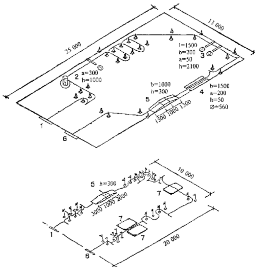
Площадки для слалома на креслах-колясках
