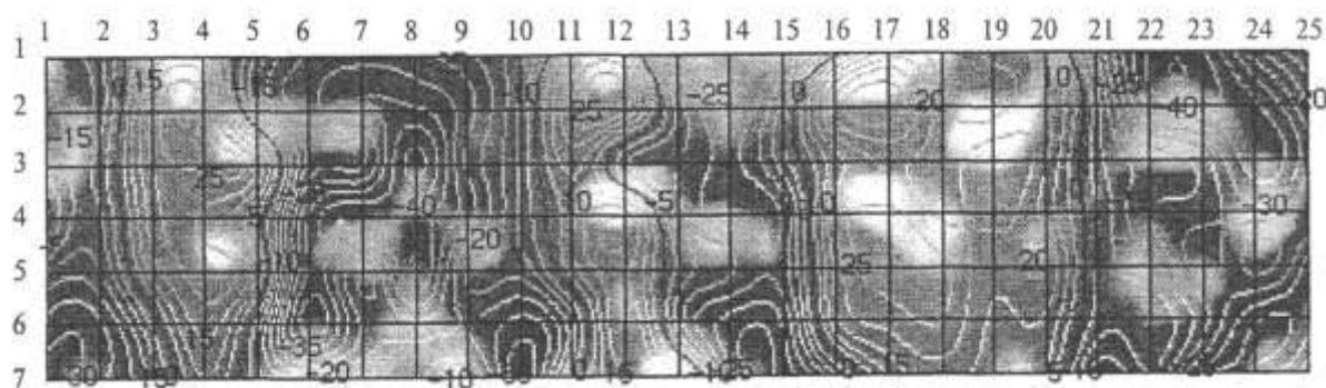
Рисунок К.1 - Пример изображения карты РГМН с областями остаточных пластических деформаций (гофры) конструкции на дисплее ПЭВМ оператора (области между 2 - 5, 10 - 13 и 15 - 21 вертикальными координатными линиями, области остаточных пластических деформаций оконтурены изострессами со значением 0 - на дисплее ПЭВМ красные линии)
